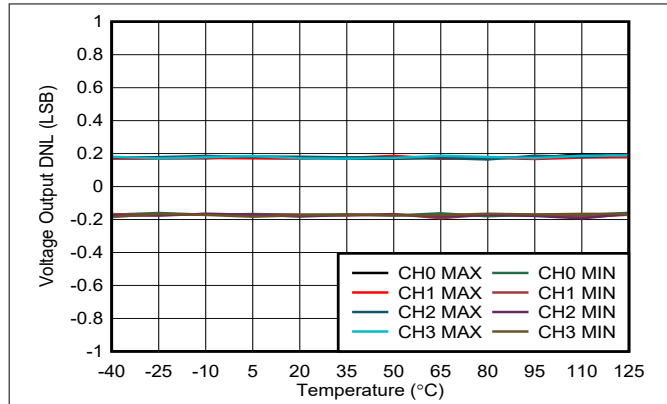
图 6-10. 电压输出 DNL 与温度间的关系
