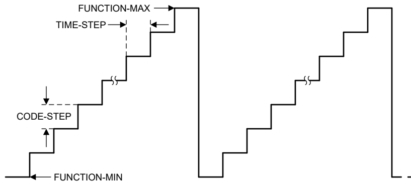
图 7-13. 锯齿波形
