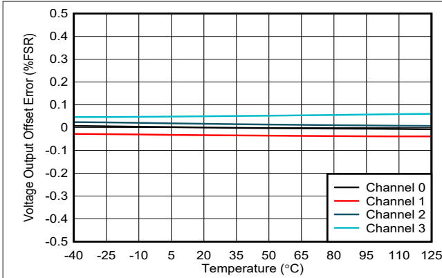
图 6-16. 电压输出偏移误差与温度间的关系
