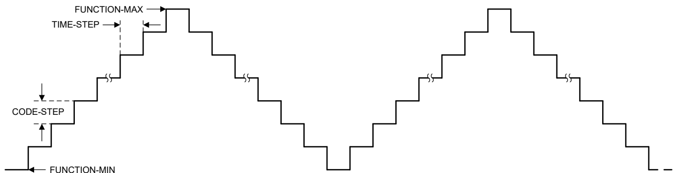
图 7-12. 三角波形
