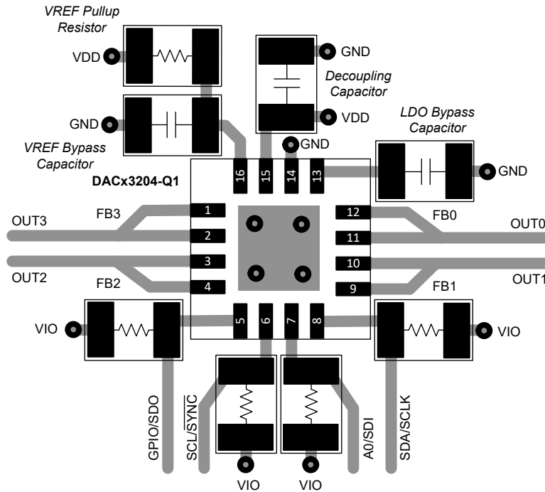
图 8-4. 布局示例
