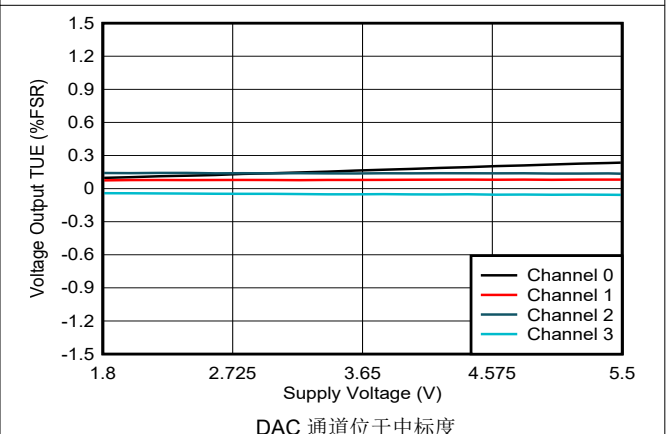
图 6-15. 电压输出 TUE 与电源电压间的关系
