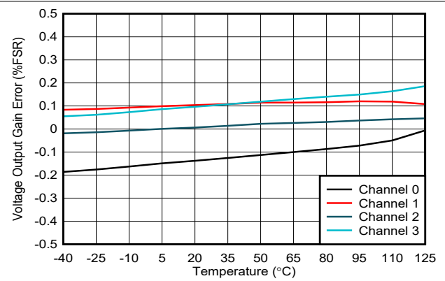
图 6-17. 电压输出增益误差与温度间的关系
