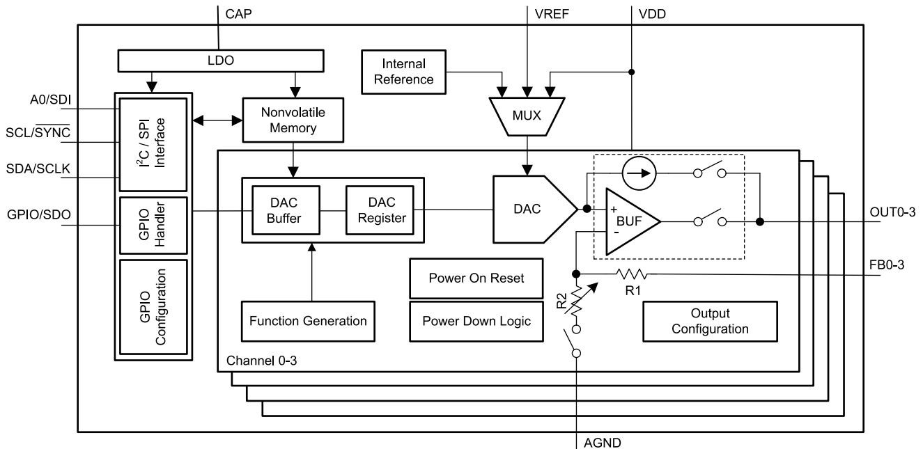
图 7-1. 功能方框图
