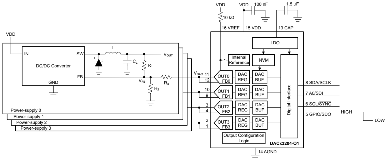
图 8-1. APD 偏置
